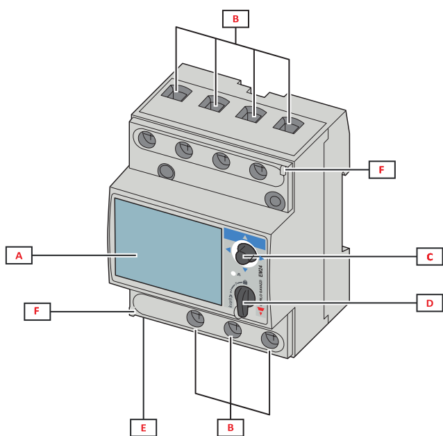
Fig. 1 Direkte tilslutning
